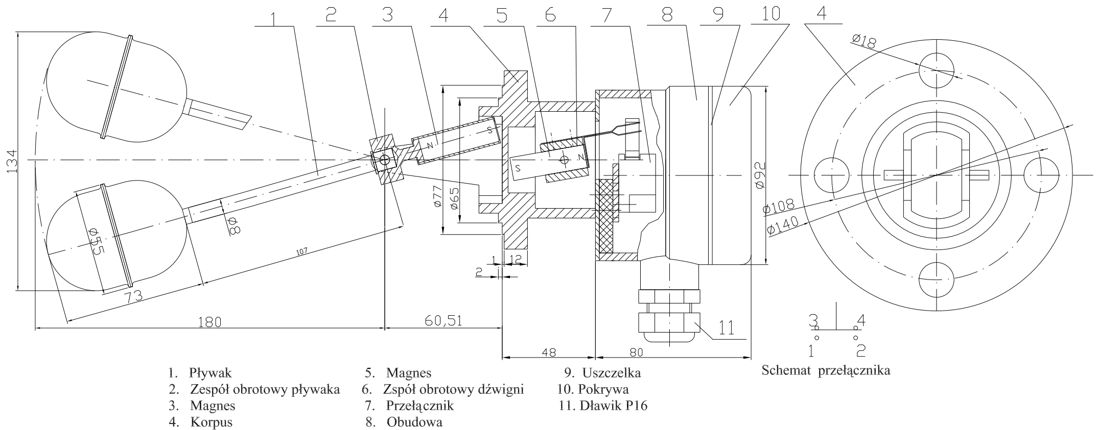
Rys.1. Pływakowy sygnalizator poziomy PSP-1.1-O-1-P-1-2,5-1-1-1
